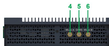
Vue de dessus d'un Box PC Optimized
