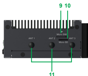
Vue de dessous de Harmony BX1
