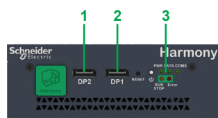
Vue de face d'un Box PC Optimized
