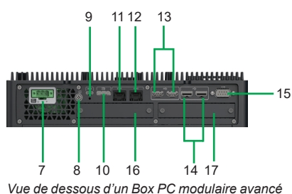
Vue de dessous d'un Box PC modulaire avancé
