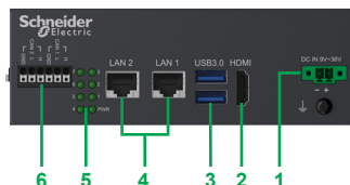
Vue de face de Harmony BX1
