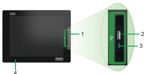
Vue de face HMIDM6 4:3
