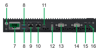
Vue de dessous de la Box Atom Harmony
