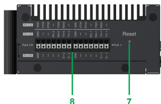
Vue de dessus de Harmony BX1
