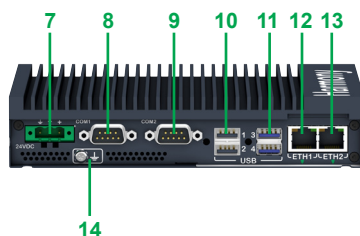
Vue de dessous d'un Box PC Optimized, version standard
