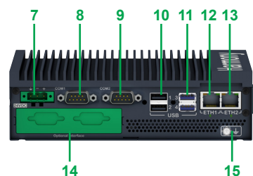
Vue de dessous d'un Box PC Optimized, version extensible
