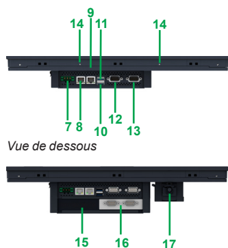
Vue de dessous avec kit d'extension
