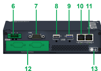
Vue de dessous d'un Box PC Basic
