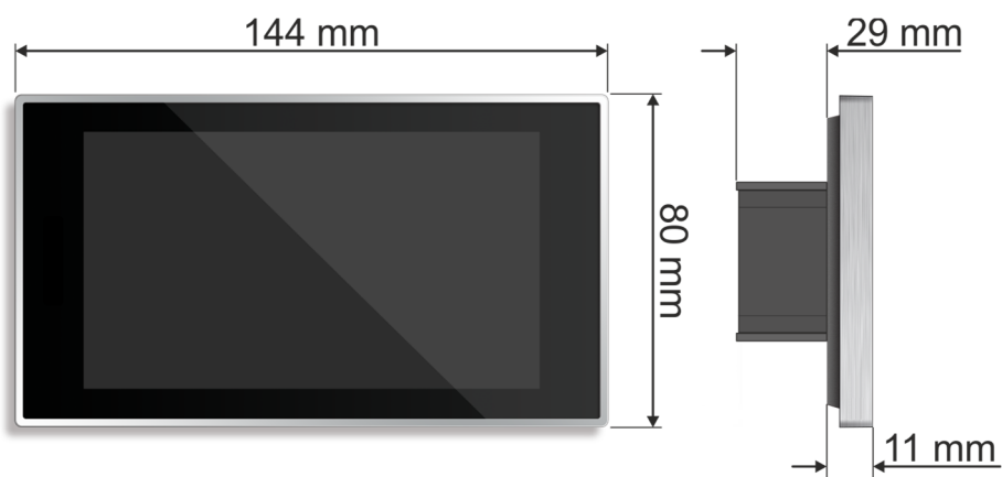
Afb. 4: Afmetingen
