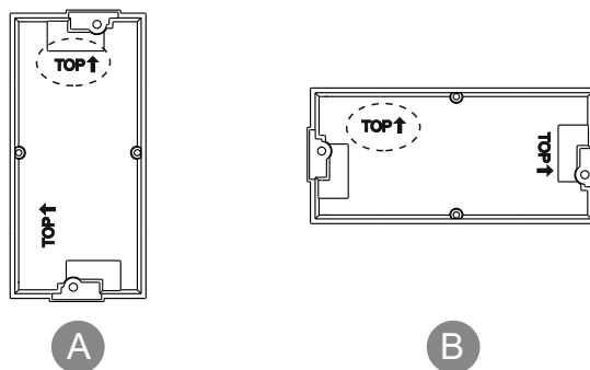
Afb. 8: Inbouwmontagedoos Oriëntatie/markering
