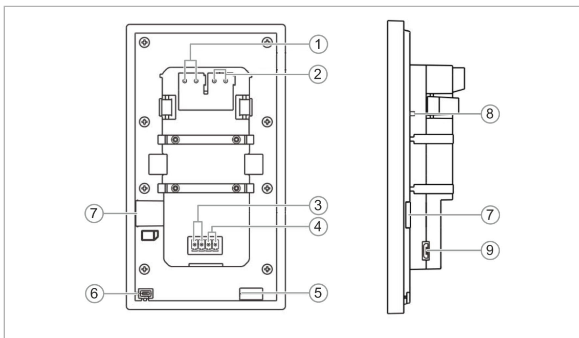
Afb. 3: Apparaatoverzicht achterzijde Busch-RoomTouch® 5, inbouw
