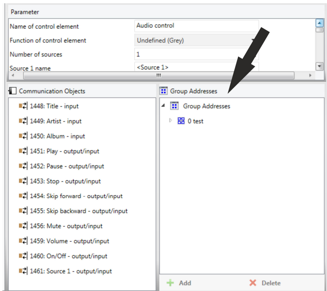
Afb. 30: Deel "Groepsadressen"
