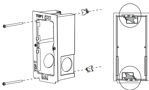
Afb. 11: Bevestigingsklemmen monteren
