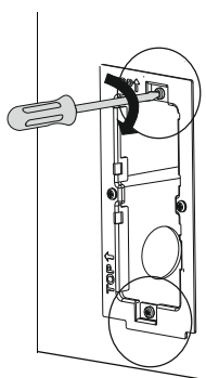
Afb. 13: Hollewandoos bevestigen
