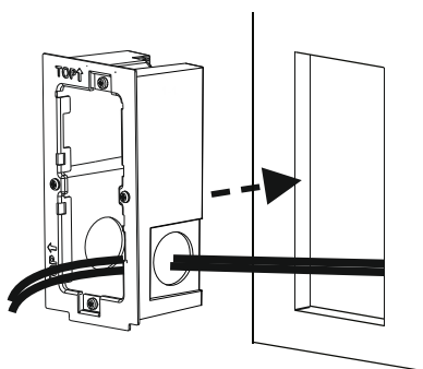
Afb. 12: Kabel invoeren
