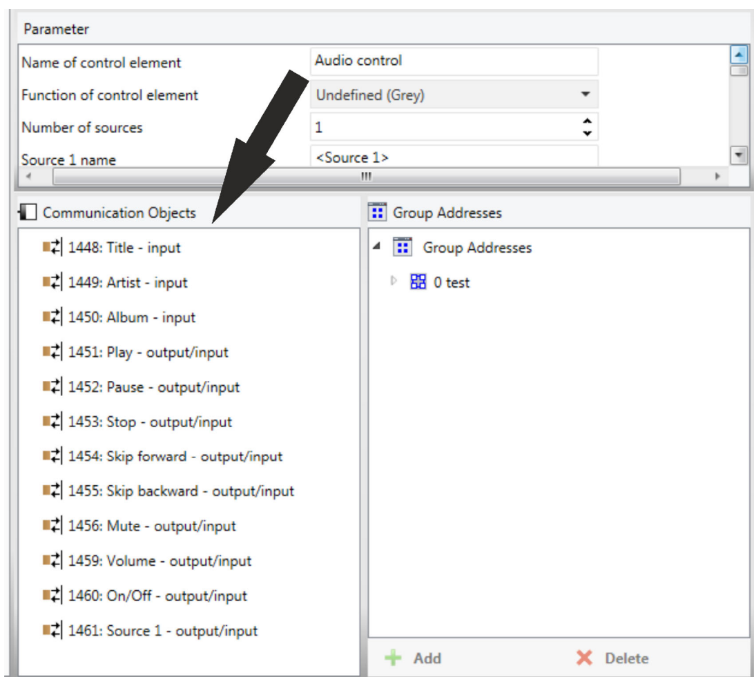
Afb. 29: Deel Communicatieobjecten
