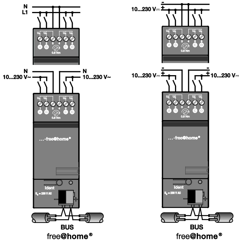
Abb. 11: Elektrischer Anschluss 6241/4.0
