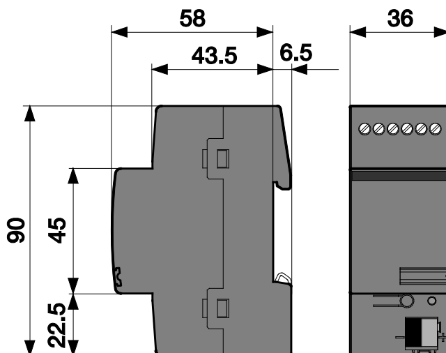
Abb. 8: Abmessungen 6241/4.0
