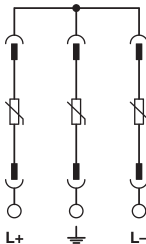
schakelschema
