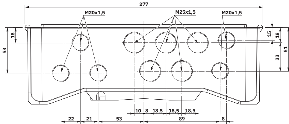
Maatschets
