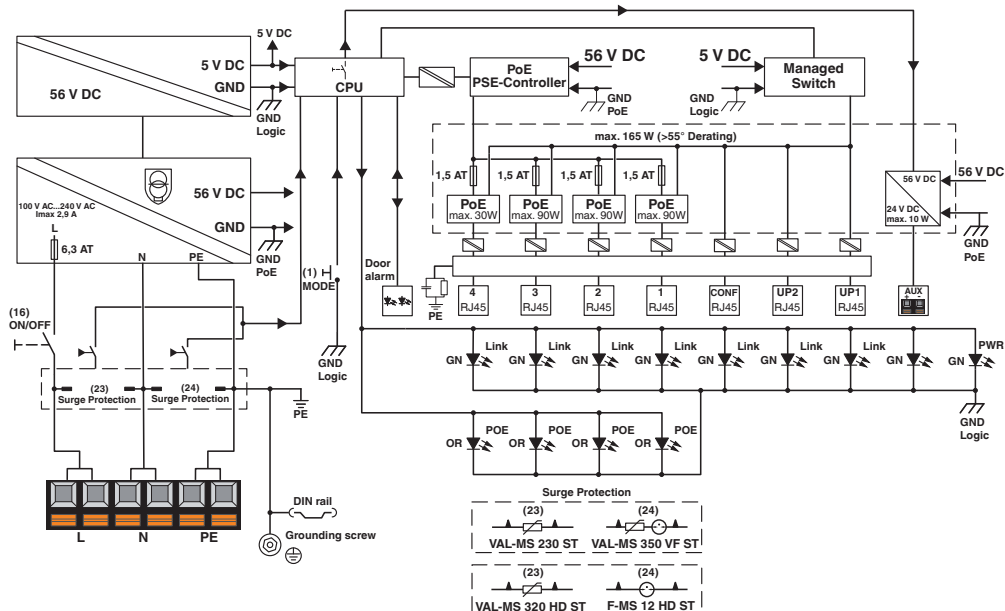
schakelschema
