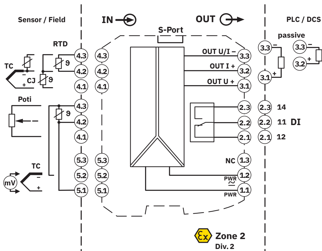
blokschema
