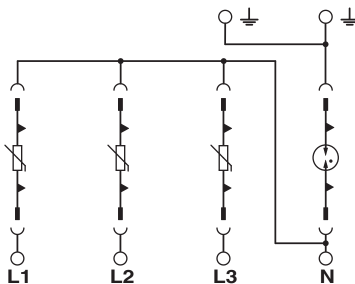
schakelschema
