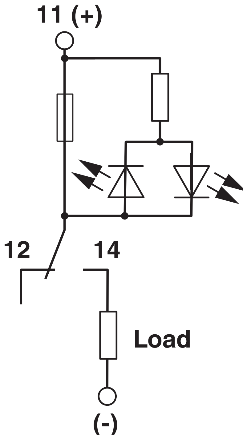
schakelschema
