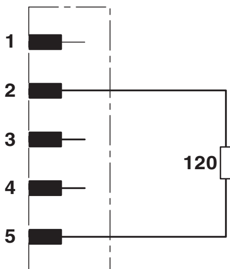
schakelschema
