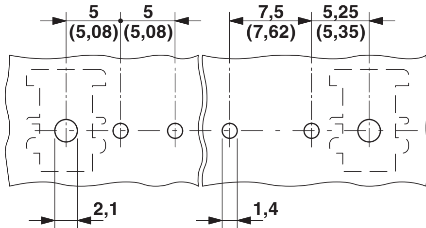
boorsjabloon/soldeerpadgeometrie
