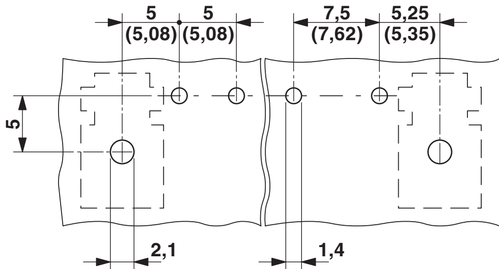
horizontaal liggend basiselement
