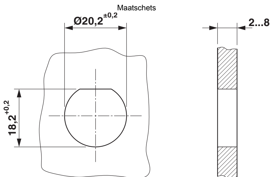
Maatschets van de QPD W 5x2,5 M20
