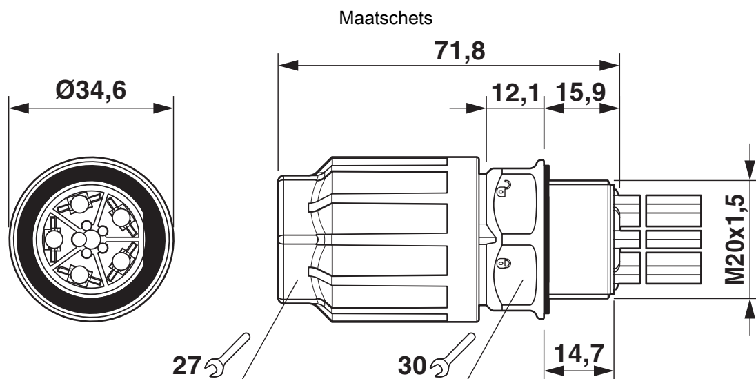
Maatschets van de QPD W 5x2,5 M20
