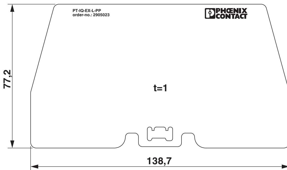
Maatschets
