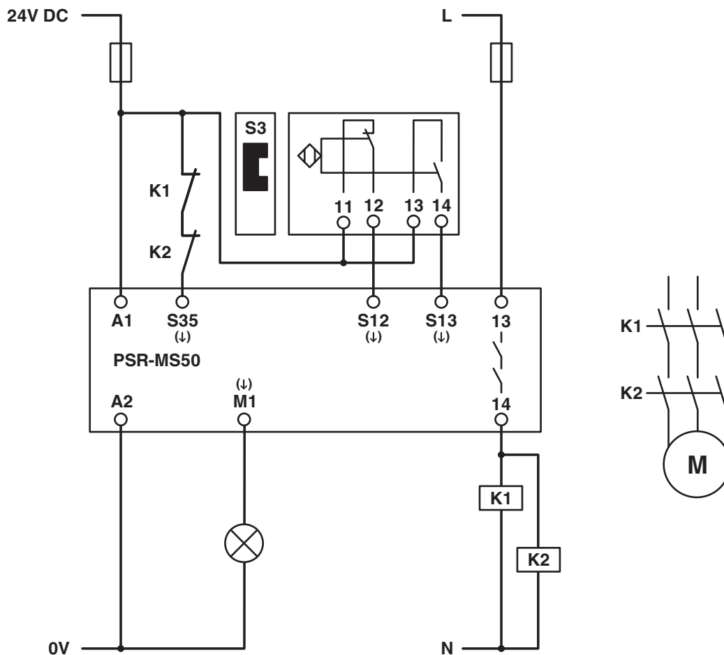
schakelschema
