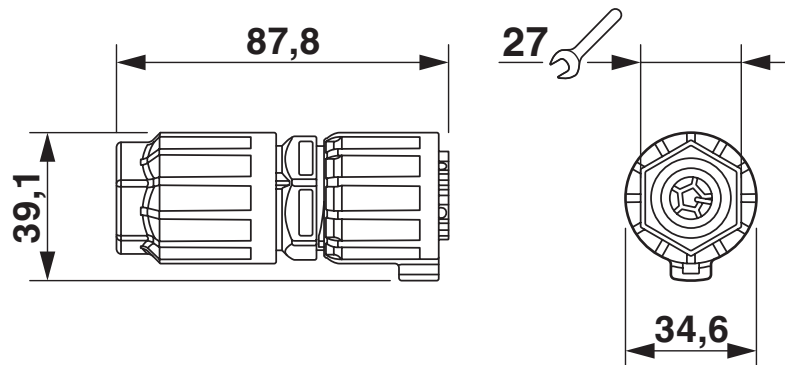
Maatschets
