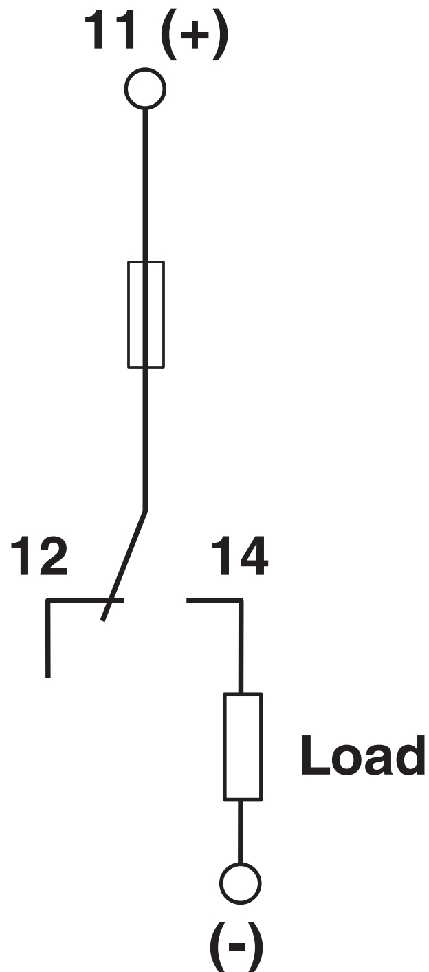
schakelschema
