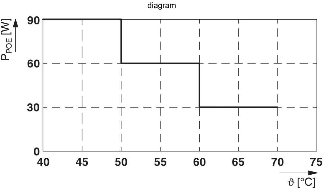
Derating (totaal PoE-vermogen)
