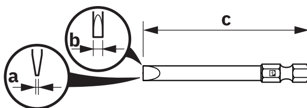
Maatschets
