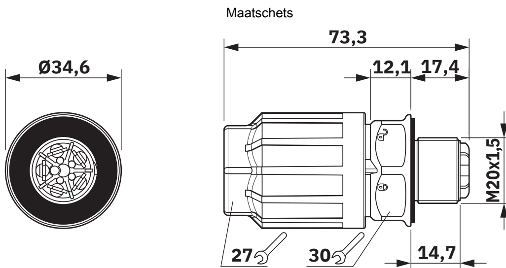
Maatschets van de QPD W 5x2,5 M20
