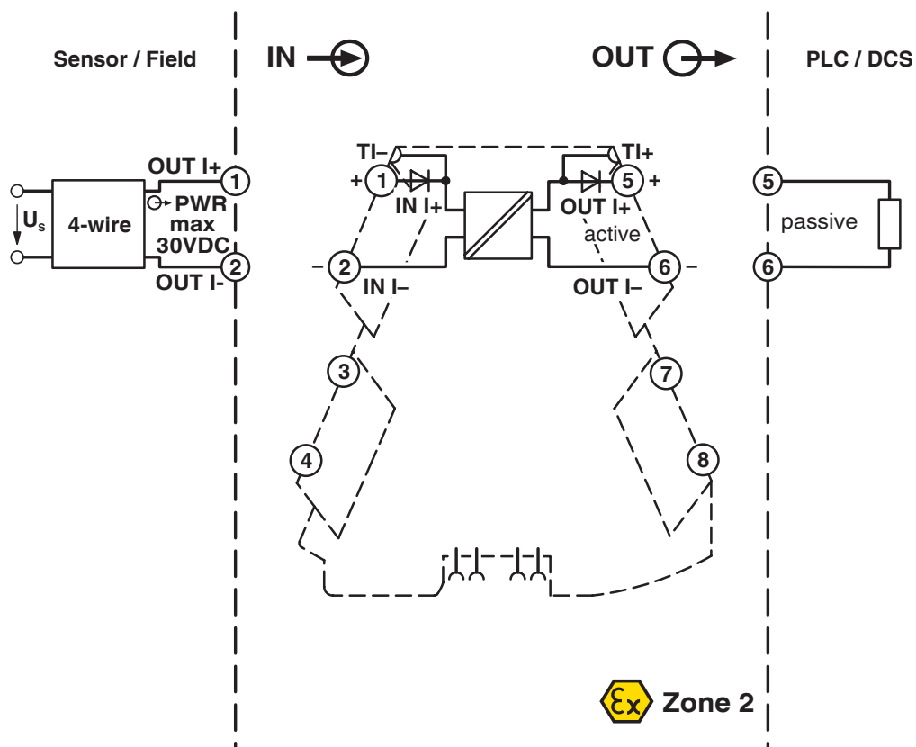
blokschema
