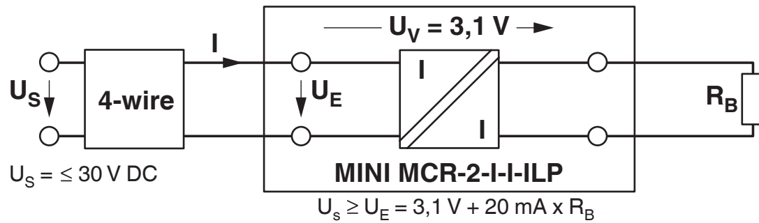
applicatietekening
