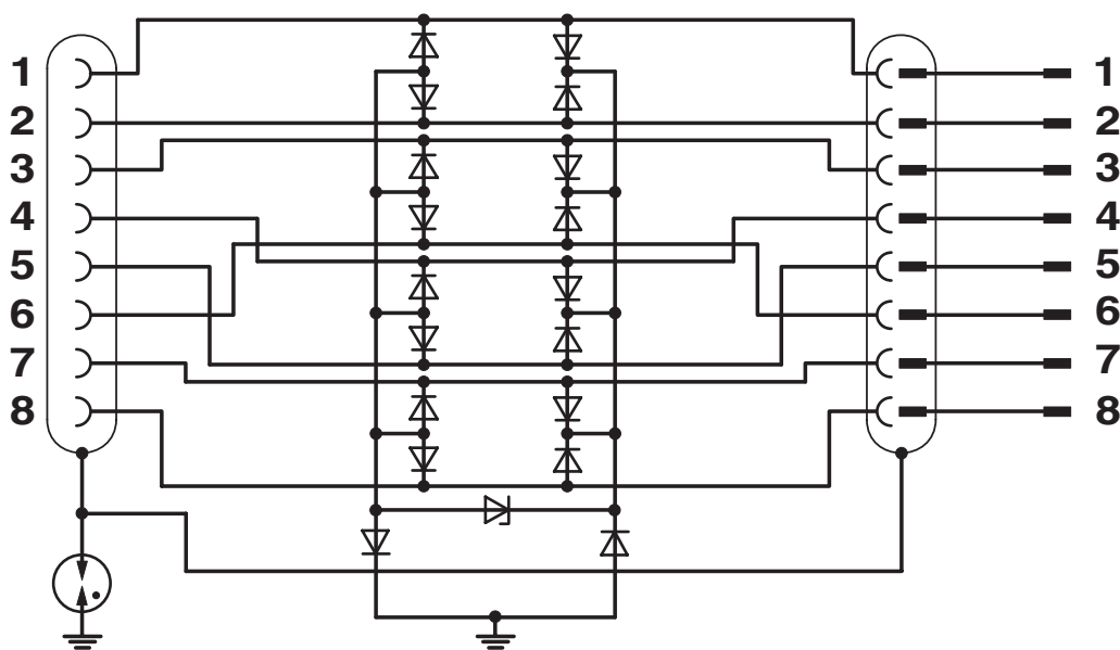
schakelschema
