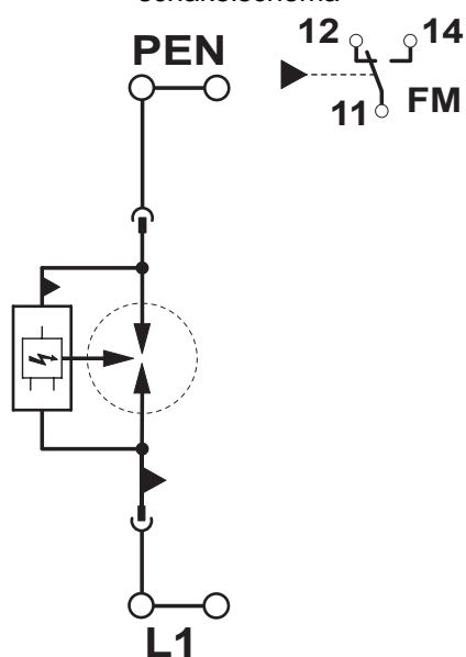
schakelschema
