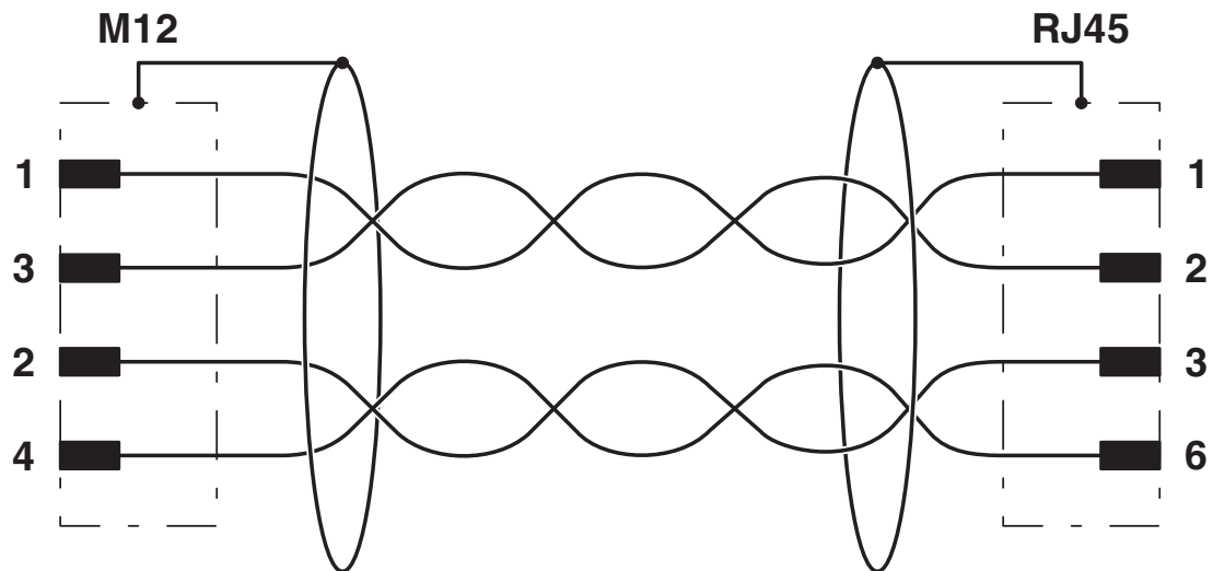
schakelschema
