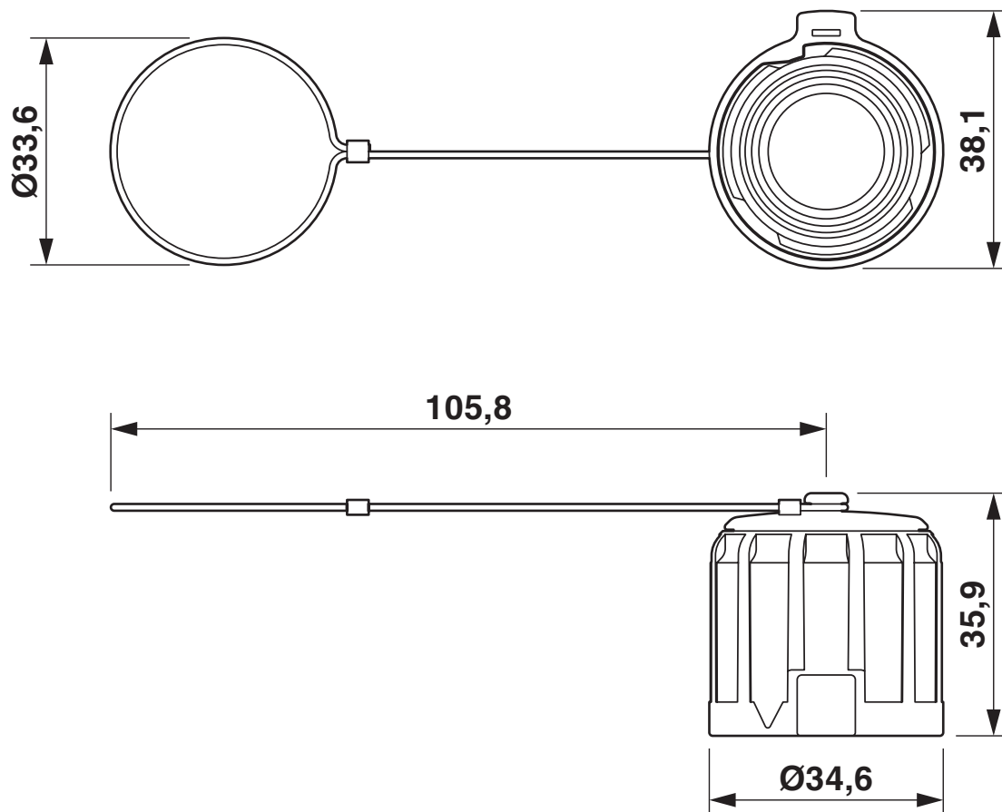
Maatschets
