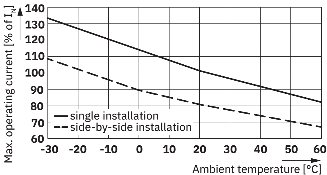
Correctiefactor bedrijfsstroom
