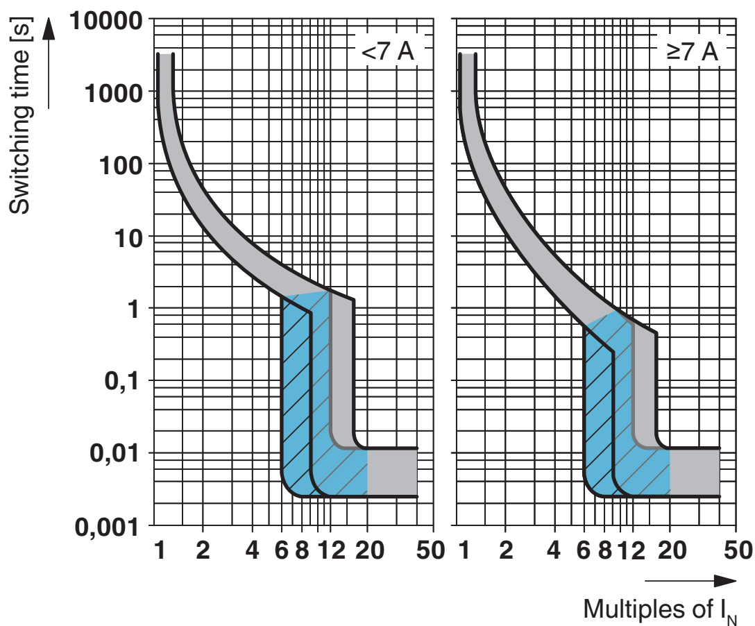
Uitschakelkarakteristiek
