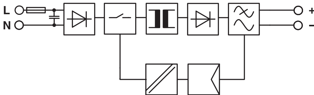
blokschema
