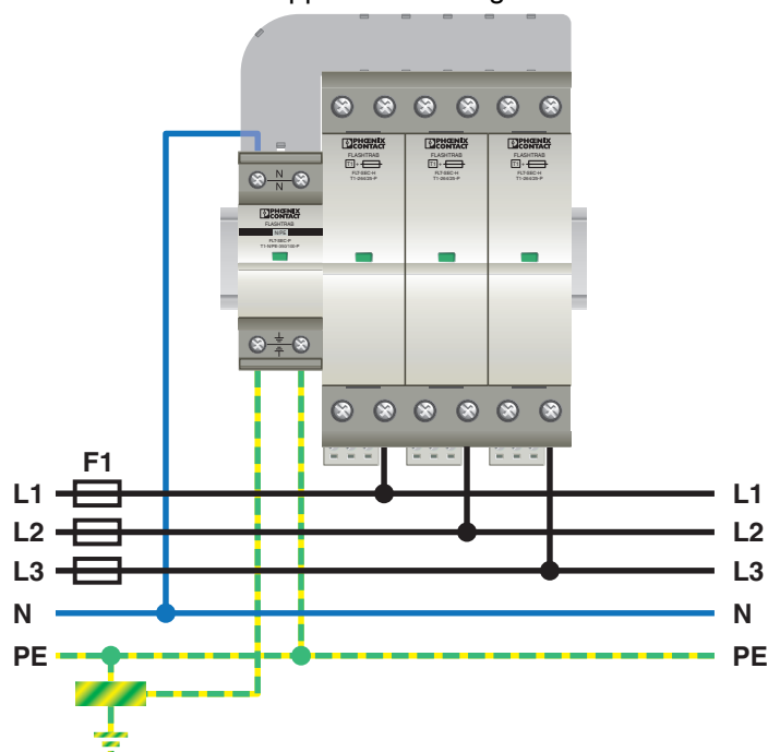
applicatietekening
