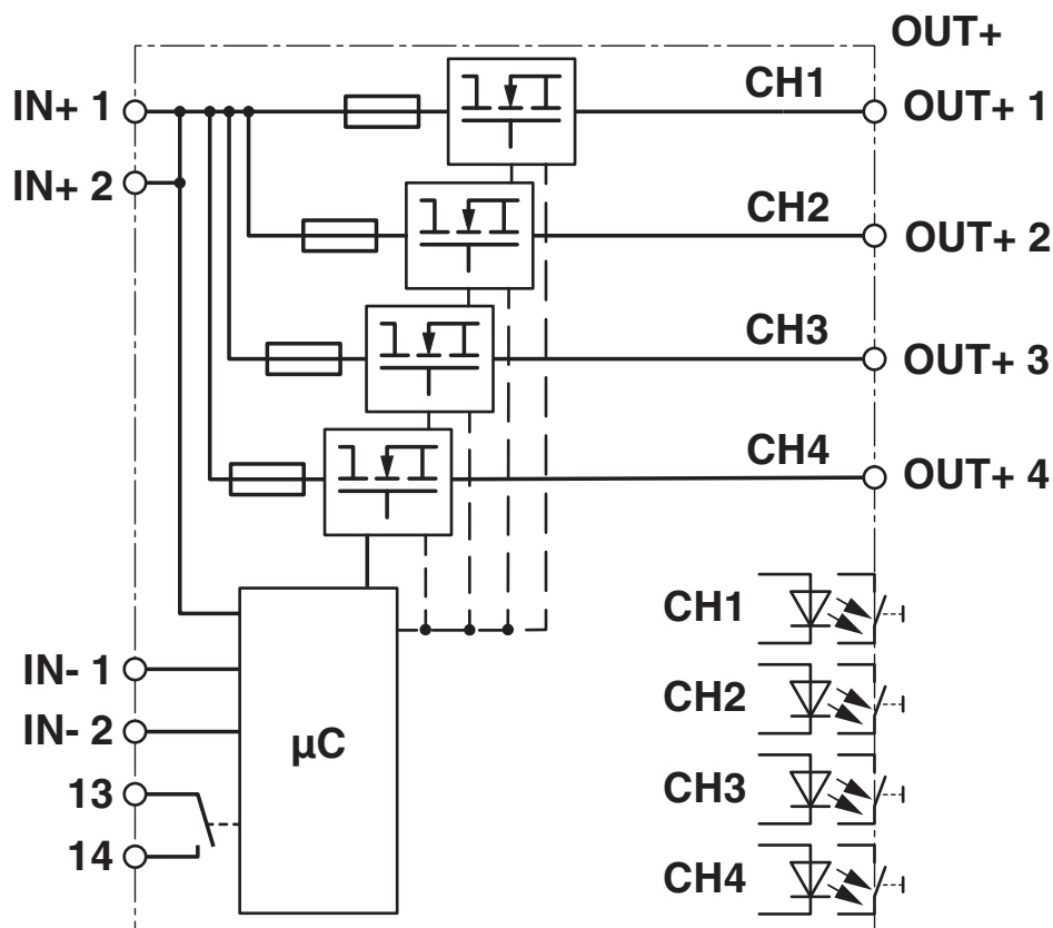
blokschema
