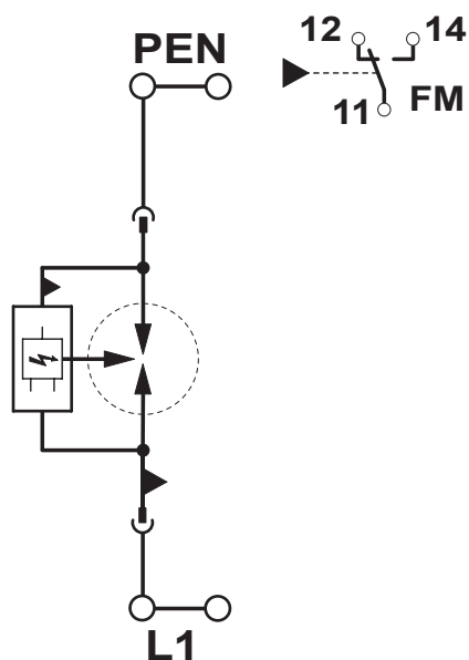
schakelschema
