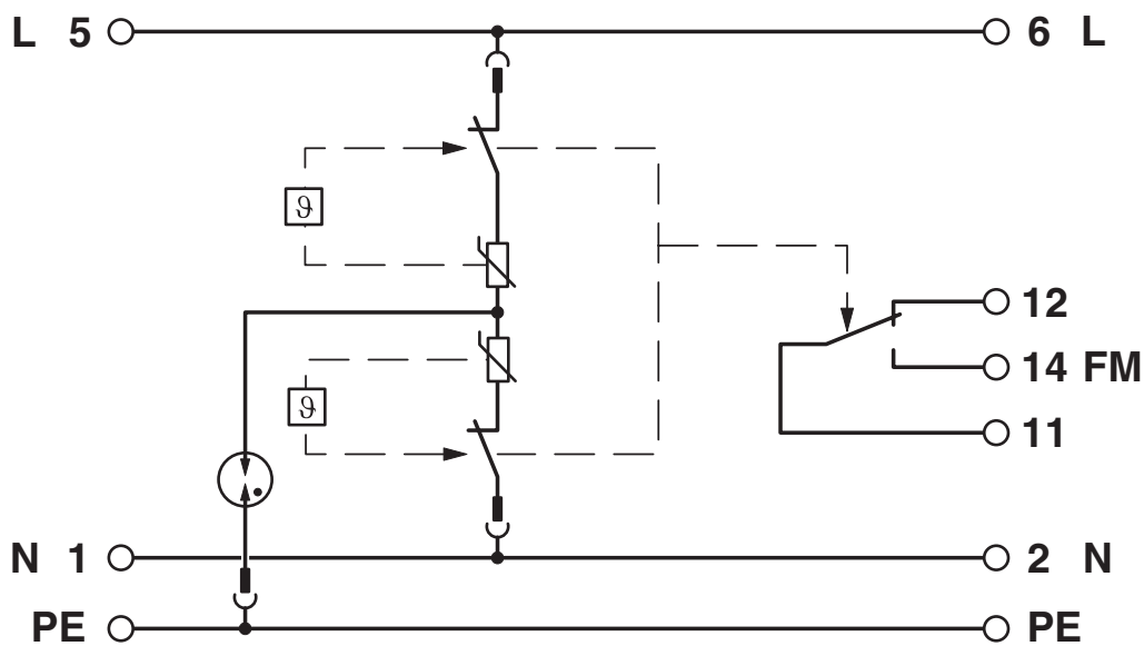
schakelschema
