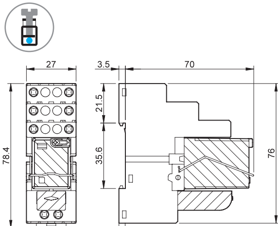
Type 58.P3 Push-in aansluiting
