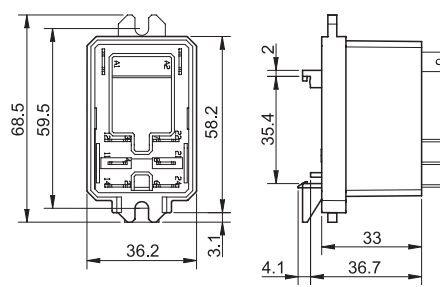
066.07 met relais
