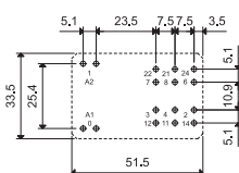
2 wisselcontacten
