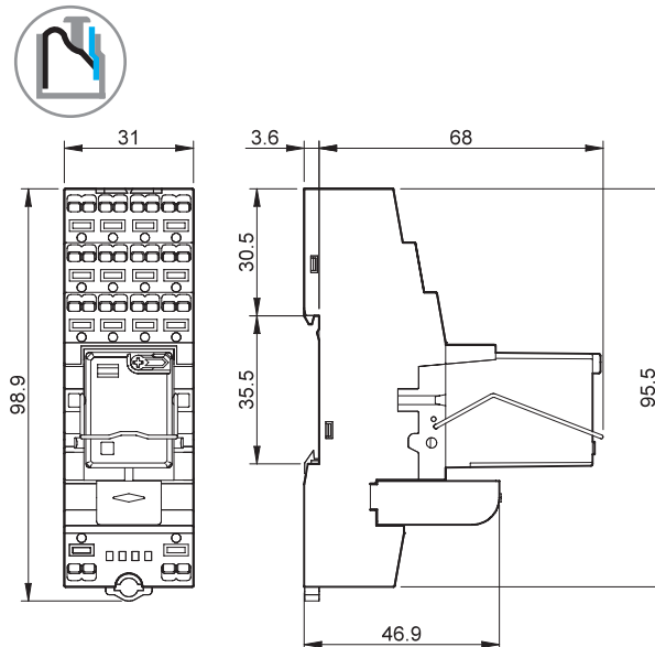
Type 58.P4 Push-in aansluiting
