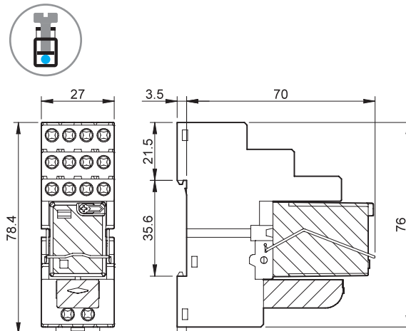
Type 58.P4 Push-in aansluiting
