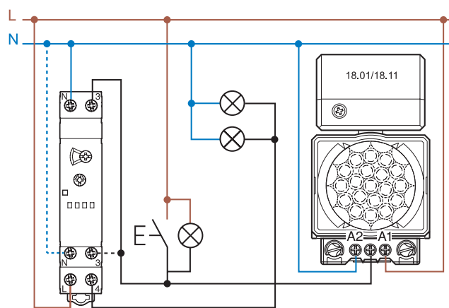
4-draads aansluiting (alleen met 18.01.8.230.0000 of 18.11.8.230.0000)
