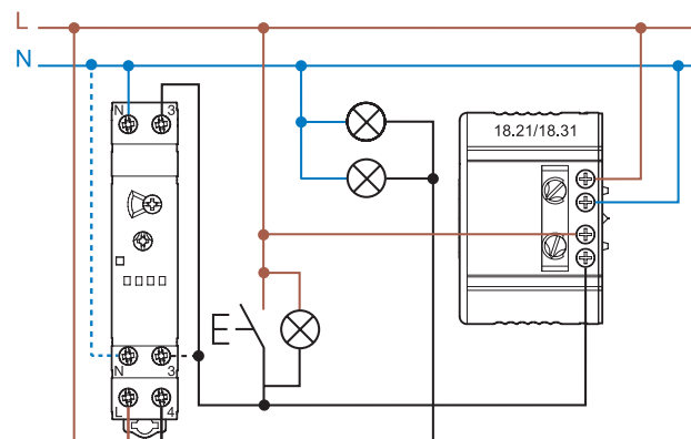
4-draads aansluiting (alleen met 18.21.8.230.0300 of 18.31.8.230.0300)
