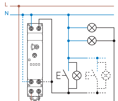
3-draads aansluiting (N verbonden met drukknop)*
