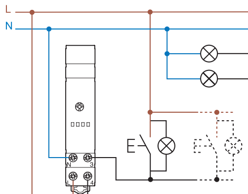
4-draads aansluiting (L verbonden met drukknop)
