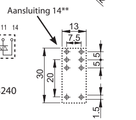
95.15.2 Aanzicht op de aansluitingen
