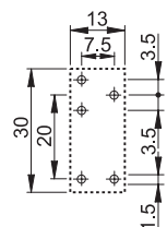
95.13.2 Aanzicht op de aansluitingen
