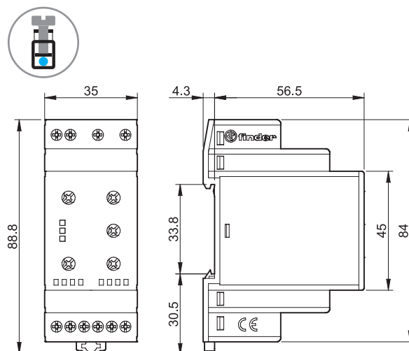
Type 70.42 Kooiklemmen
