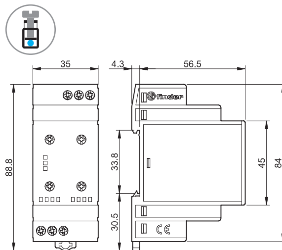
Type 70.31 Kooiklemmen
