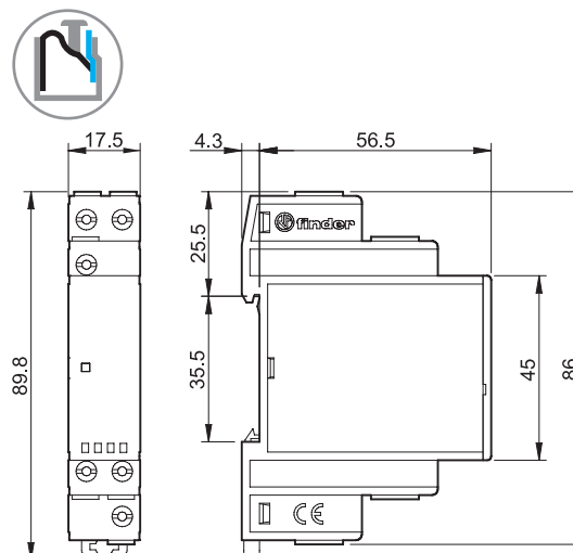
Type 70.61-P000 Push-in aansluiting
