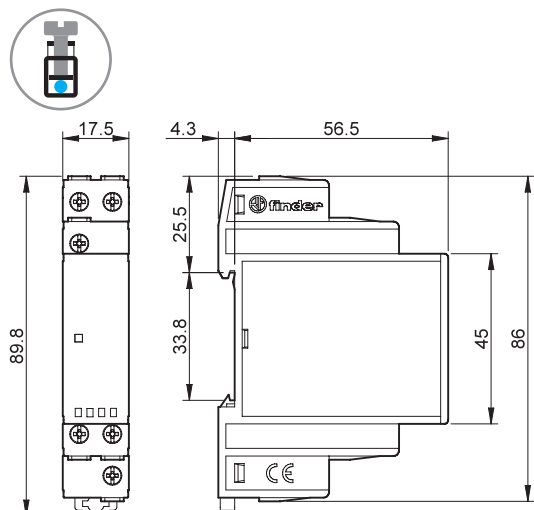
Type 70.61 Kooiklemmen
