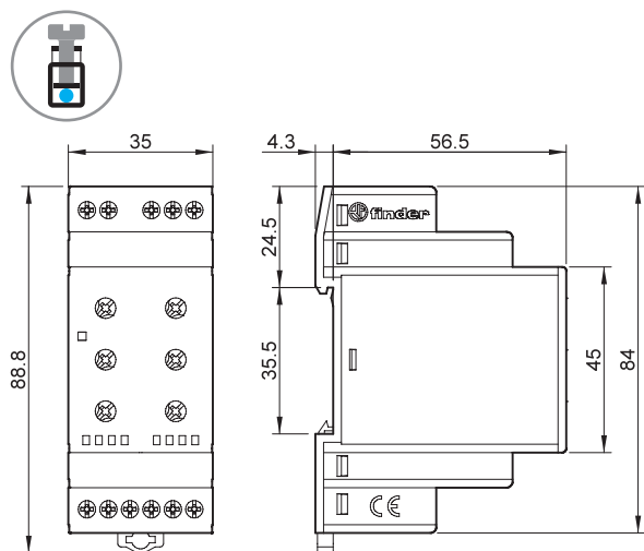
Type 70.61 Kooiklemmen
