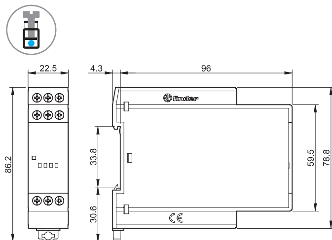
Type 70.62 Kooiklemmen
