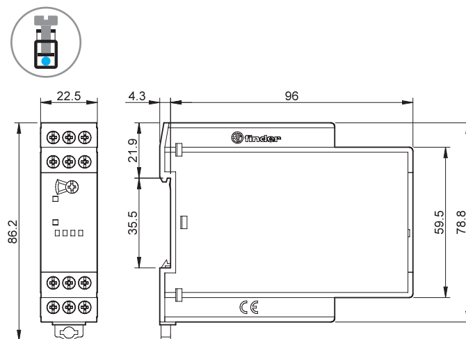
Type 70.92 Kooiklemmen
