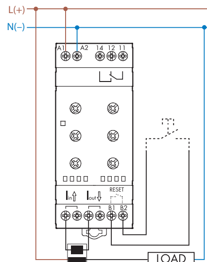
Type 70.51 Werking met omvormer
