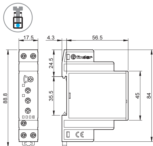
Type 70.11 Kooiklemmen
