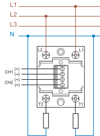
2-fasen aansluiting (77.x2)
