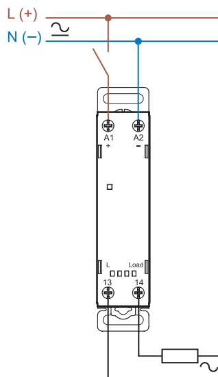
1-fase aansluiting (77.31...805x)
