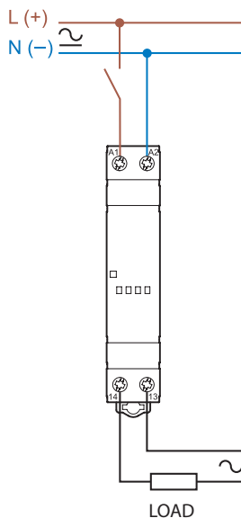
1-fase aansluiting (77.31...805x)
