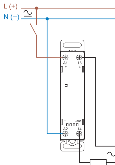
1-fase aansluiting (77.31...807x)
