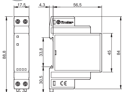
Type 77.x2 Centraalschroefklem
