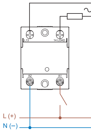
1-fase aansluiting (77.x1)
