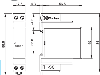
Type 77.01 DC Kooiklemmen
