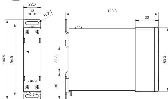
Type 77.x1 Centraalschroefklem
