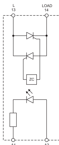
Principeschakeling
