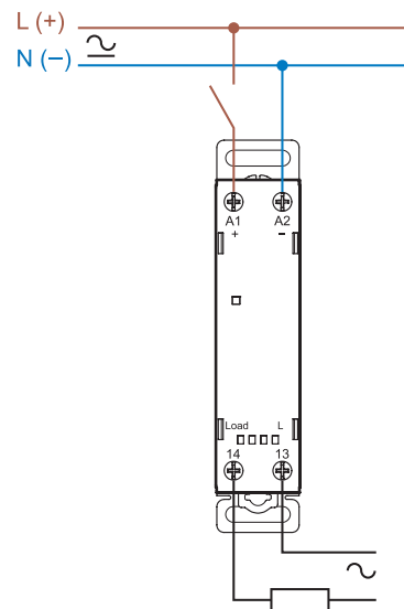
1-fase aansluiting (77.11/77.21)
