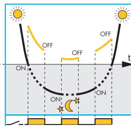
Traditionele schemeringsschakelaar met beïnvloeding door de geschakelde verlichting
