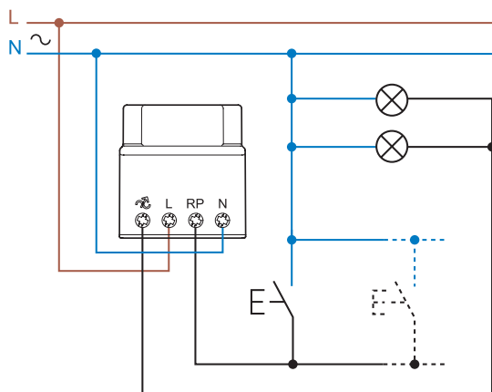
Type 15.81 - 3-draads aansluiting (N verbonden met drukknop)
