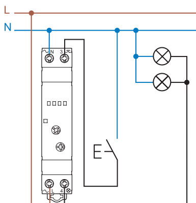
Type 15.81 - 3-draads aansluiting (N verbonden met drukknop)
