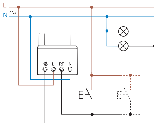
Type 15.81 - 4-draads aansluiting (L verbonden met drukknop)
