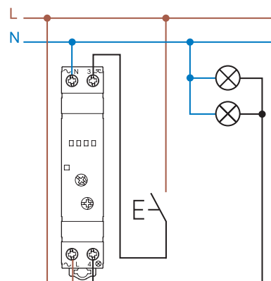
Type 15.81 - 4-draads aansluiting (L verbonden met drukknop)
