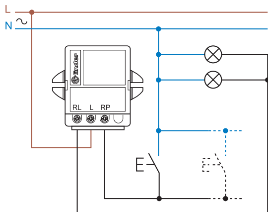
Type 15.91 - 3-draads aansluiting (N verbonden met drukknop)
