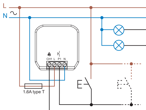
Type 15.21 - 4-draads aansluiting
