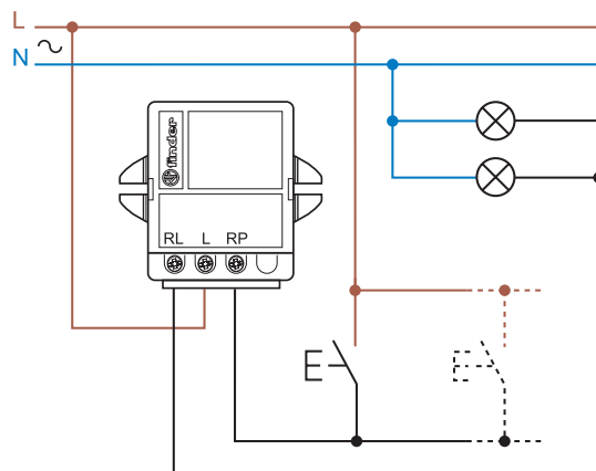
Type 15.91 - 4-draads aansluiting (L verbonden met drukknop)
