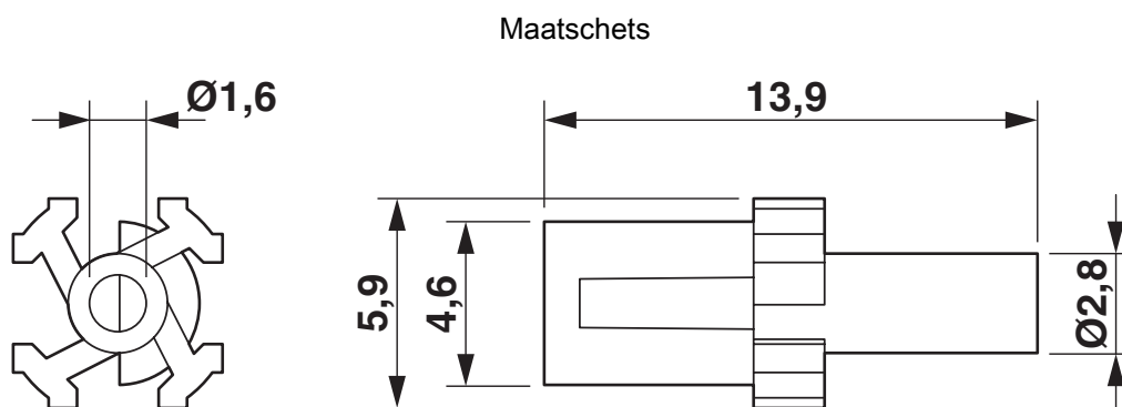
schematekening
