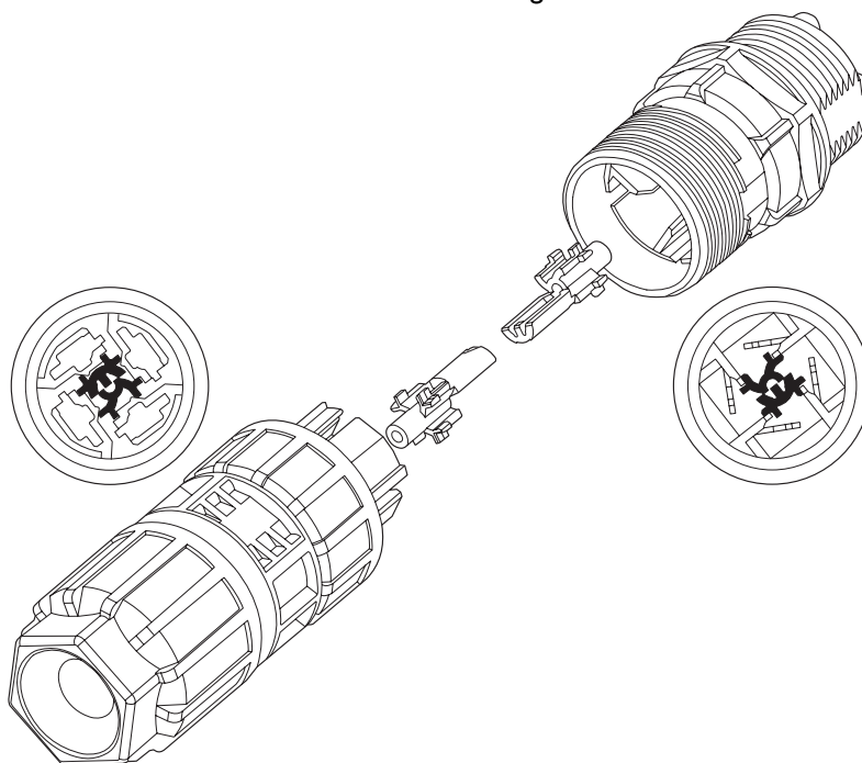
schematekening
