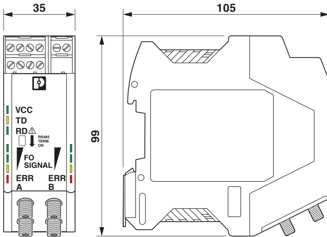
Maatschets
