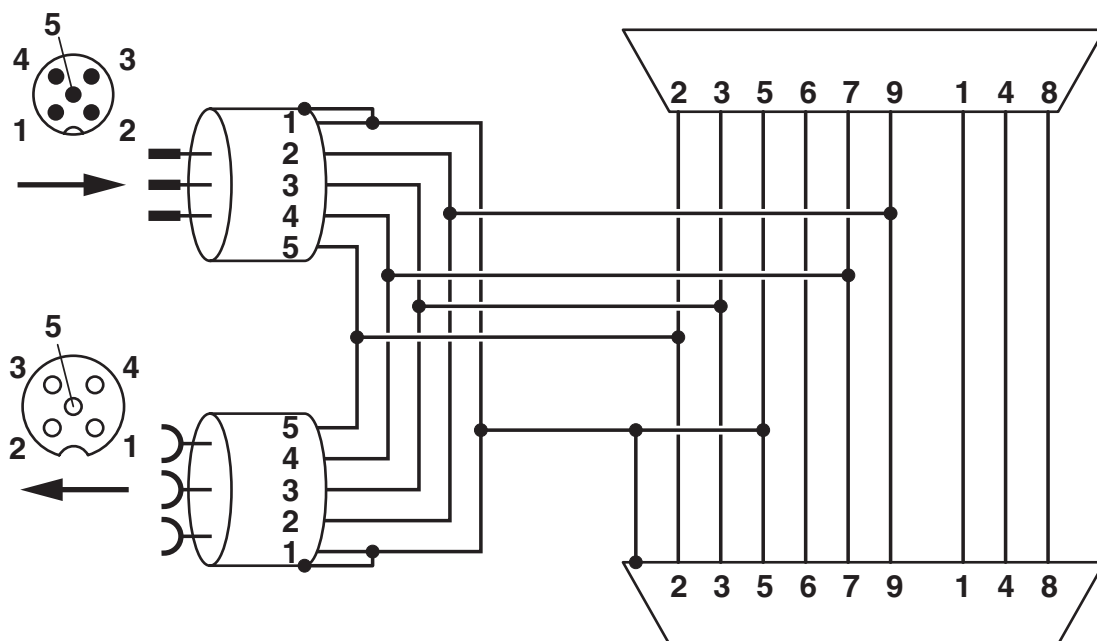
Functieschakelschema SUBCON-PLUS-CAN/...M12
