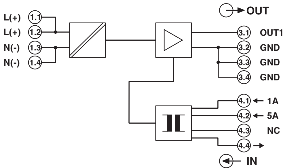
schakelschema
