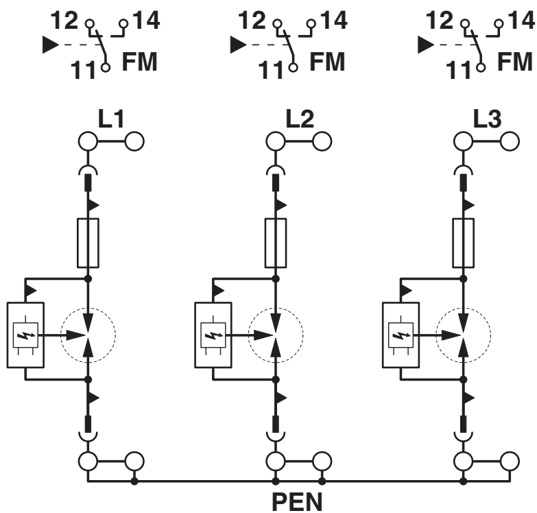
schakelschema
