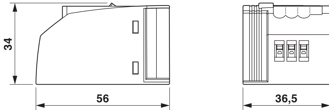
Maatschets
