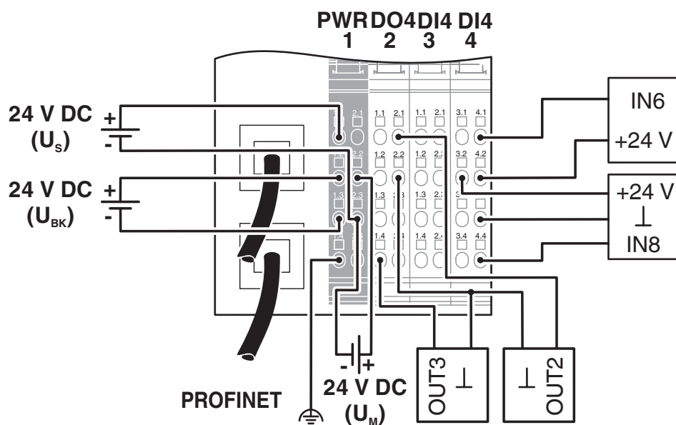
aansluitschema
