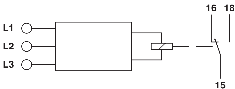
blokschema
