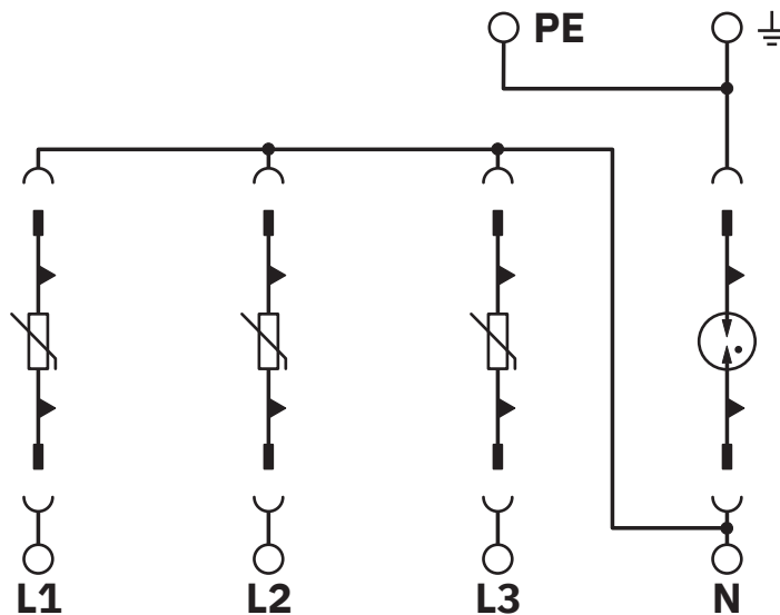
schakelschema
