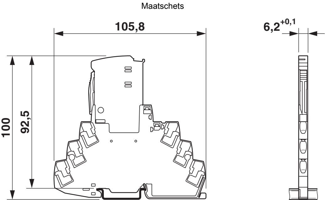
schematekening
