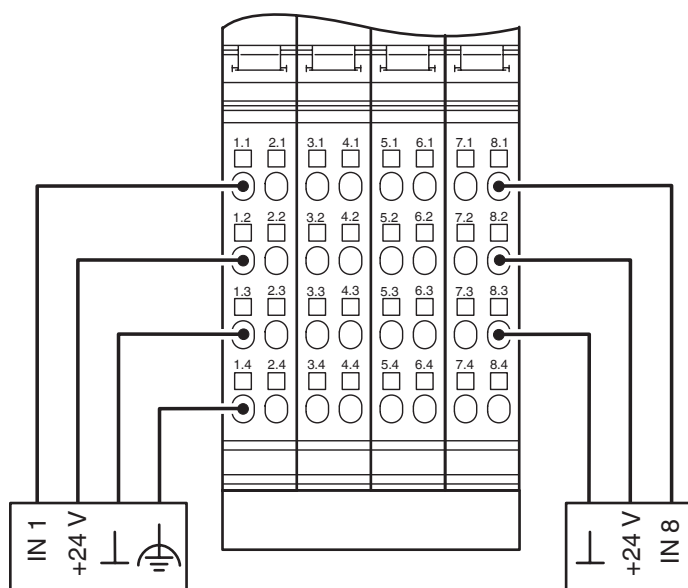
aansluitschema
