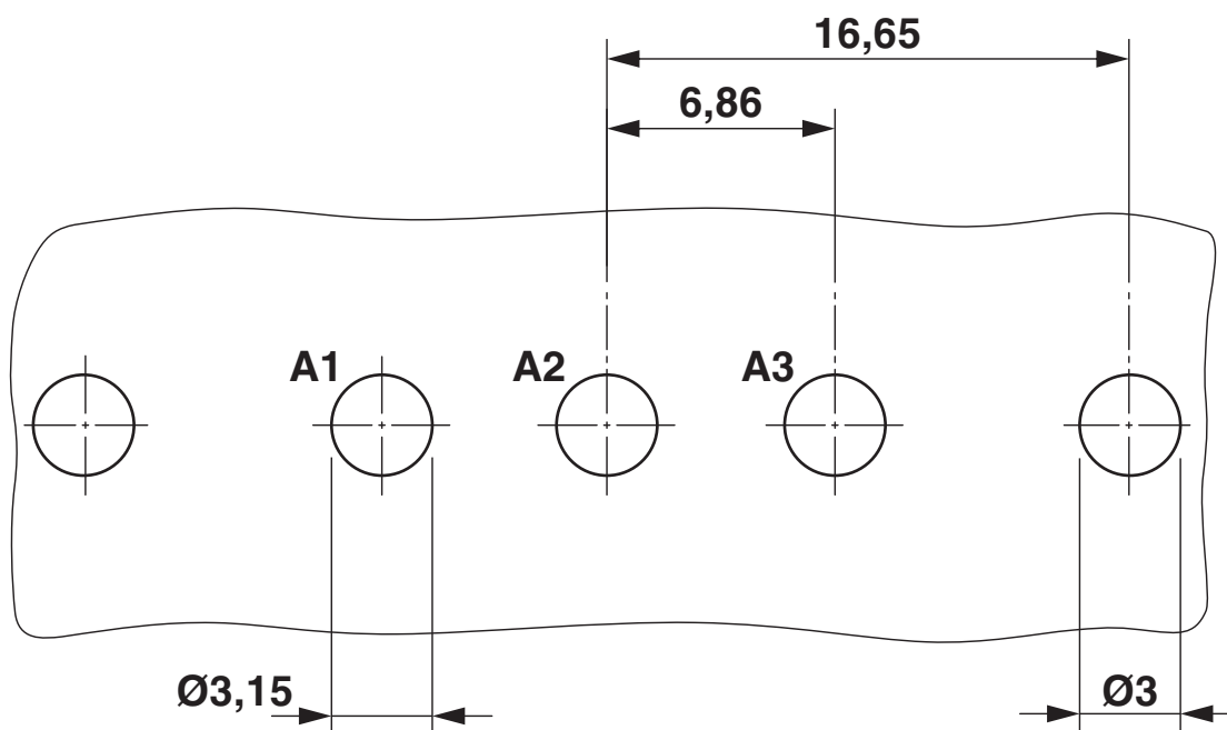
boorsjabloon/soldeerpadgeometrie
