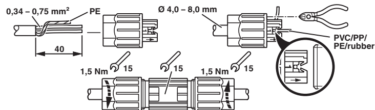
functietekening
